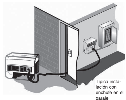
Generador enchufado en la entrada de alimentación intercambiable de un interruptor de transferencia por medio de un cordón de 7.6 metros (25 pies) (Instalación Posible con Accesorios Reliance Disponibles)
