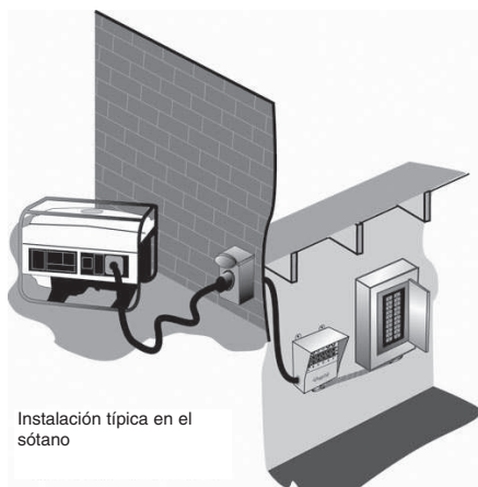
Generador enchufado en un tomacorriente exterior, conectado por cable a un interruptor de transferencia instalado cerca del centro de carga en el sótano. (Instalación Posible con el Juego)
