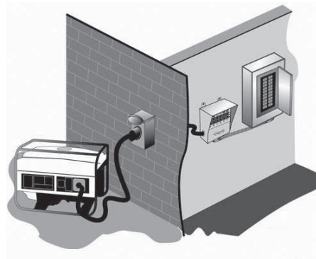
Generador enchufado en un tomacorriente exterior, conectado por cable a un interruptor de transferencia instalado cerca del centro de carga en el garaje. (Instalación Posible con el Juego)
